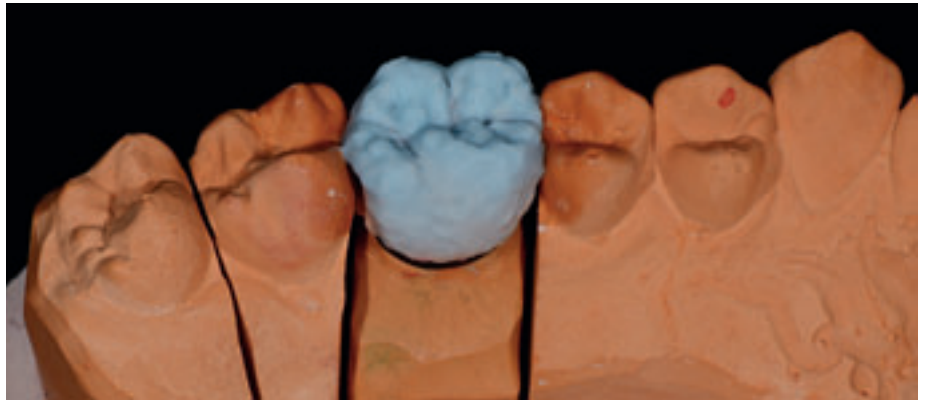
Eine mit Keramikrohmasse geschichtete Krone vor dem Brand
